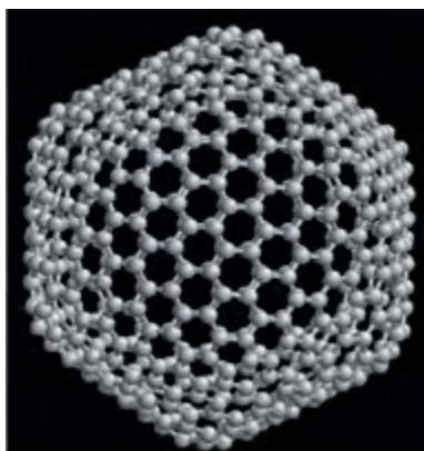
Фуллерен C50, имеющий форму икосаэдра
