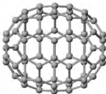
Фуллерен C70 эллипсоидный
